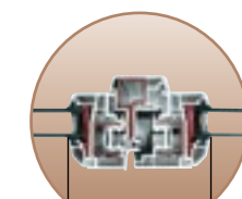
← Flügel/Stulp 7093/7303
